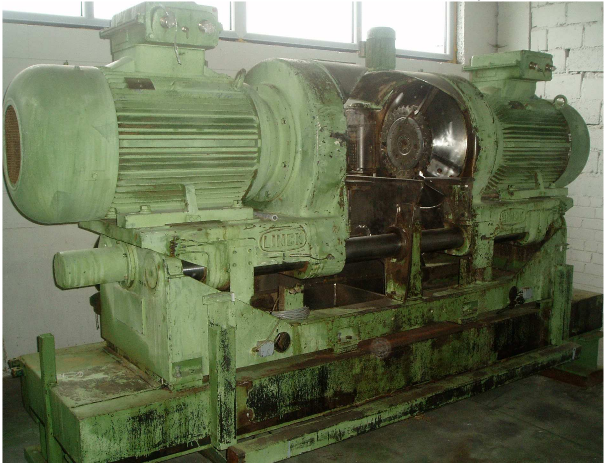
2 Stück Linck - Spaner V 18 mit jeweils 2 x 85 kW Antriebsleistung / 2 pcs. Linck canter Type V 18 with 2 x 85 kW each
